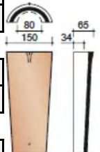
Хребтовая черепица полукруглая
