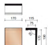
Пультовая моночерепица 90°
