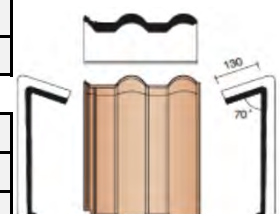
Пультовая моночерепица
