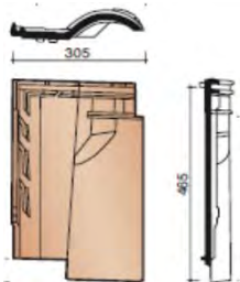
Вентиляционная черепица
