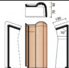
Боковая пультовая моночерепица правая
