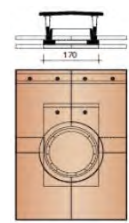
Проходной комплект для вентиляции (D=100мм)
