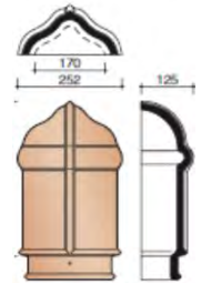
Начальная хребтовая черепица Standard
