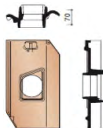
Проходная черепица для вентиляции (D=100мм)
