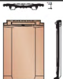
Двухволновая черепица
