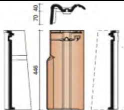
Боковая черепица левая
