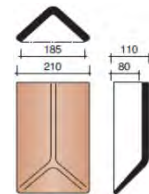
Вальмовая черепица (для хребта bonnet)
