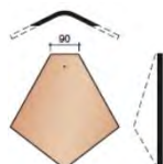
Хребтовая черепица угловая
