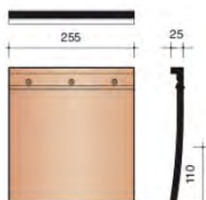
Черепица 3/2
