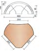
Вальмовая черепица
