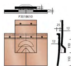
Вентиляционный комплект
