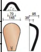
Начальная хребтовая черепица угóльная малая
