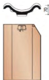
Двухволновая черепица
