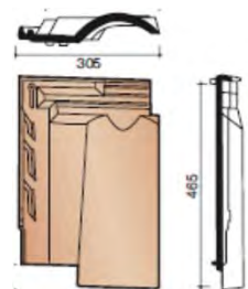
Подконьковая черепица
