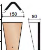
Хребтовая черепица угóльная малая
