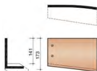
Боковая черепица 301 левая
