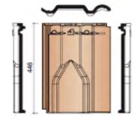
Вентиляционная черепица
