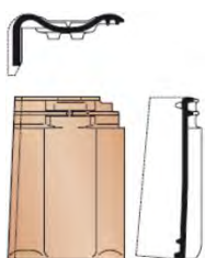
Боковая черепица левая
