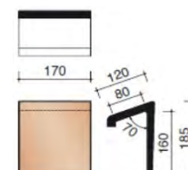
Пультовая моночерепица 70°
